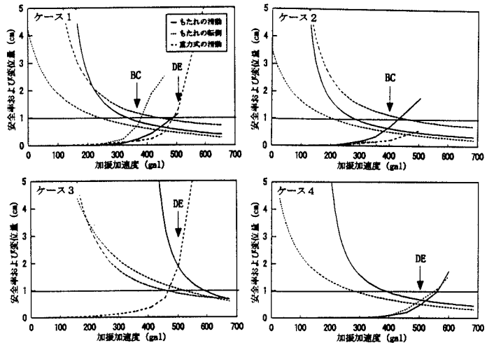
図-3 加振加速度と安全率・変位量の関係
