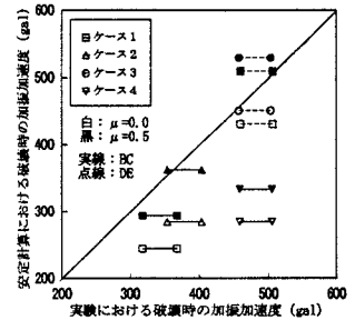
図-4 破壊加速度の比較
