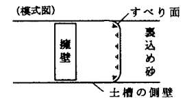
図-5 すべり面の形状
