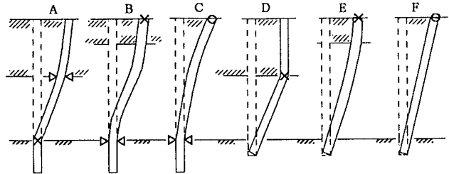
図-2 破壊パターン
