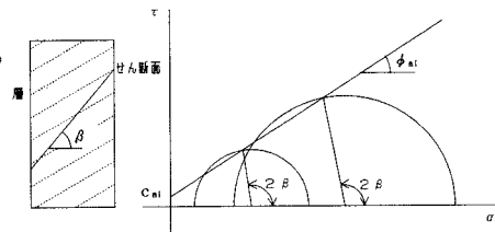
図-2 異方性を考慮した破壊線
