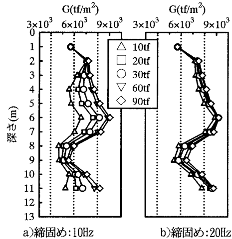
図-6 締固め加振力の効果の比較
