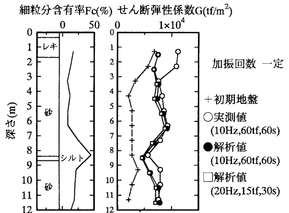
図-7 実地盤での高周波、小荷重による締固め効果
