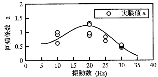
図-3 振動数と回帰係数 a の関係 せん断弾性係数 G(\text{kgf/cm}^2) せん断弾性係数 G(\text{tf/m}^2)
