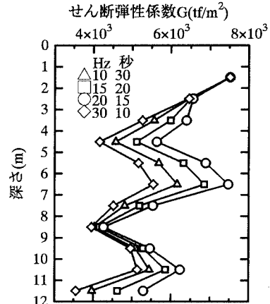
図-5 締固め振動数と加振時間の効果の比較 (WAP3による解析)
