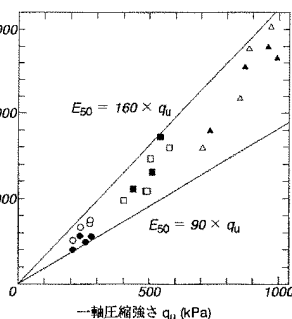
図-2 q_u \sim E_{50} 関係のまとめ
