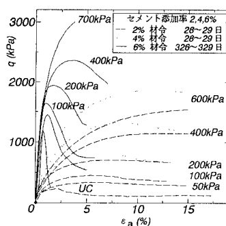
図-4. 応力～ひずみ関係
