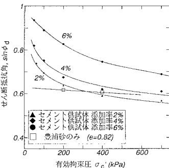
図-6. 拘束圧の増加に伴うせん断抵抗角の変化
