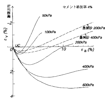
図-5. 軸ひずみと体積ひずみの関係
