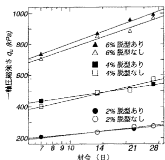
図-1 一軸圧縮強さに及ぼす材令の影響
