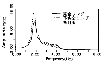
図-3 タンクトップの伝達関数
