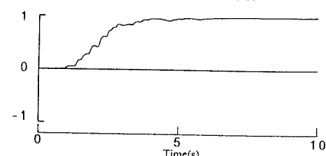
図-6 自由地盤の過剰間隙水圧比
