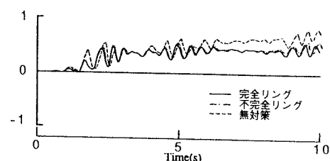
図-7 タンク中央下部地盤の過剰間隙水圧比
