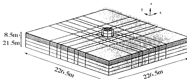
図-1 FEM解析モデル
