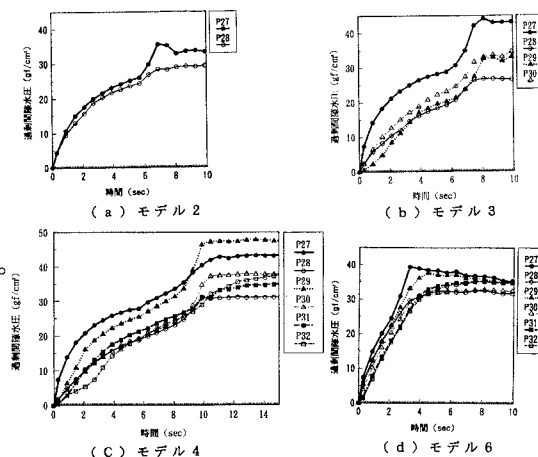
図-4. 側壁内外の過剰間隙水圧
