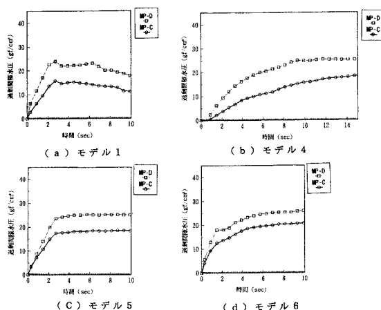
図-3. 地中構造物底板の過剰間隙水圧
