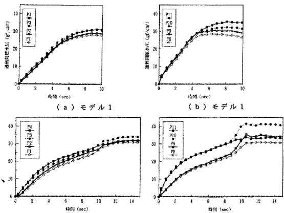
図-2. 地中構造物下の地盤の過剰間隙水圧
