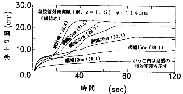
図-6 時間-浮上り量の関係（網）
