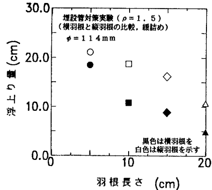
図-4 羽根長さ-浮上り量の関係
