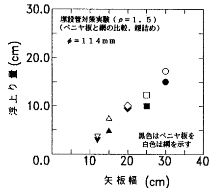
図-7 矢板幅-浮上り量の関係
