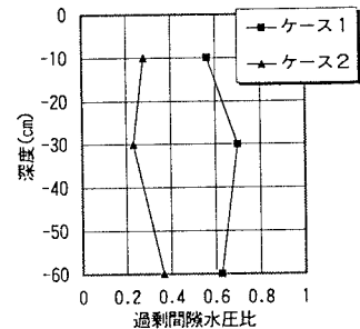
図-4 過剰間隙水圧比（レベル5、模型端部）
