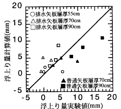
図5 浮上りの実験値と計算値の比較
