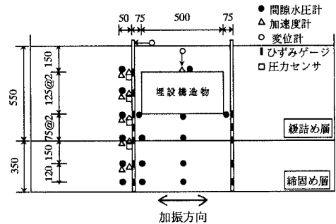
図1 実験模型と計測位置の例
