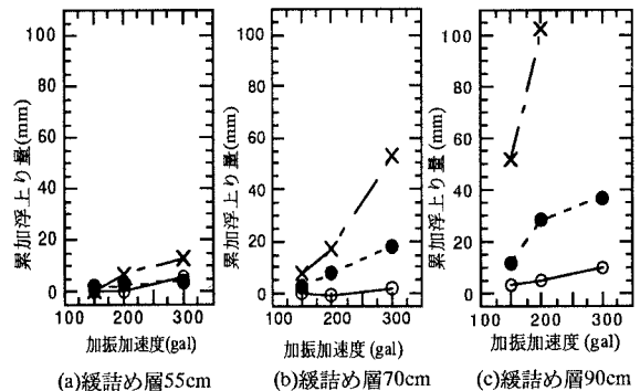
図2 累加浮上り量と加振加速度の関係
