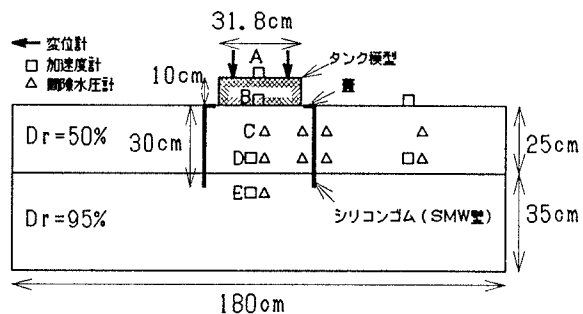
図-2 振動台実験概要
