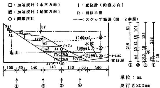
図-1 実験模型
