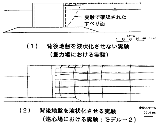
図-4 背後地盤の変形形態
