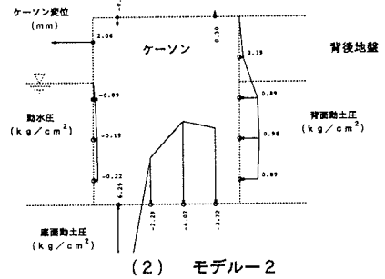
図-3 ケーソンに作用する動土圧
