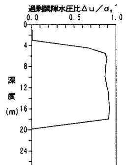
図-5 過剰間隙水圧比の分布状況
