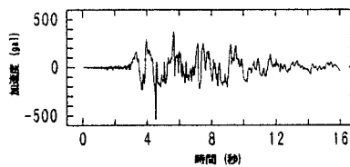
図-4 入力加速度波形 3)
