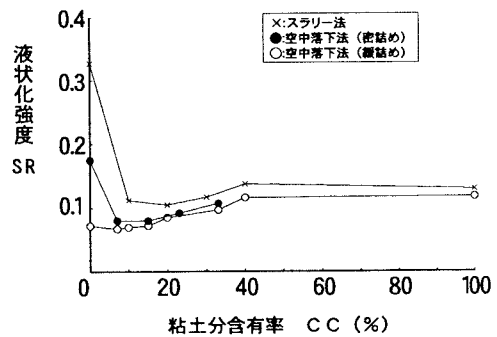
図1: 液状化強度と粘土分含有率の関係
