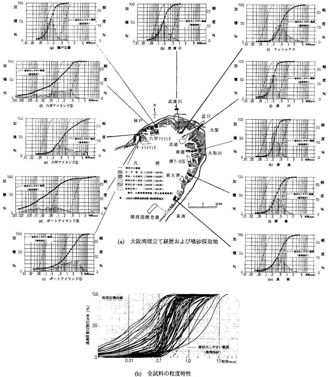
図-2 兵庫県南部地震による噴砂の粒度特性
