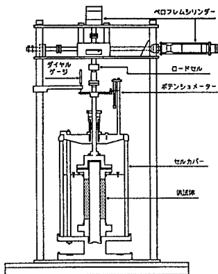
図-1 中空ねじりせん断試験機
