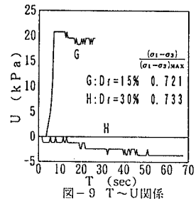
図-9 T~U関係
