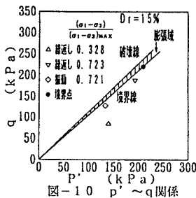
図-10 p'~q関係
