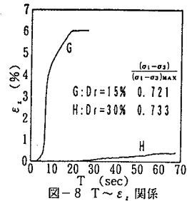
図-8 T~εv 関係
