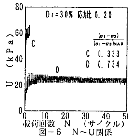
図-6 N~U関係
