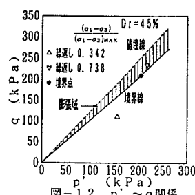
図-12 p'~q関係
