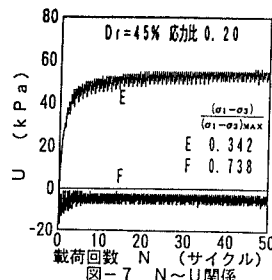
図-7 N~U関係
