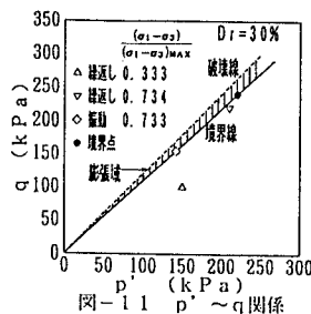
図-11 p'~q関係
