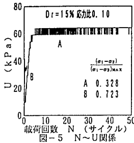
図-5 N~U関係
