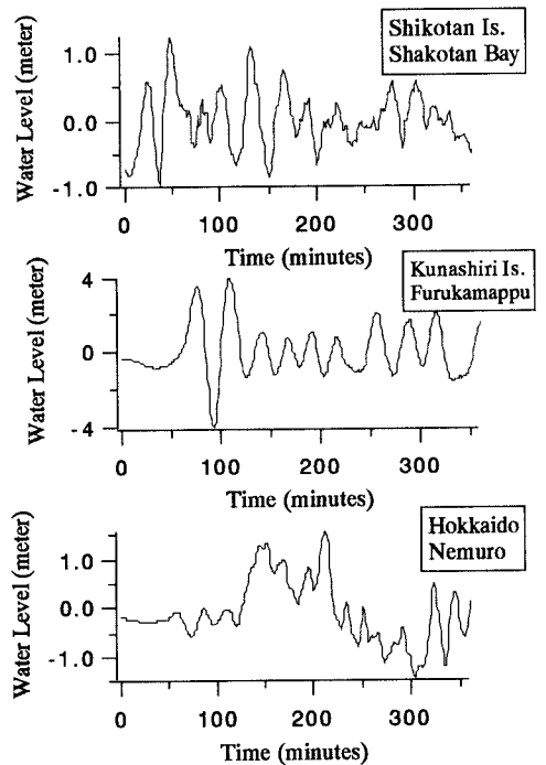
図-4 津波による水位の時間的変化
