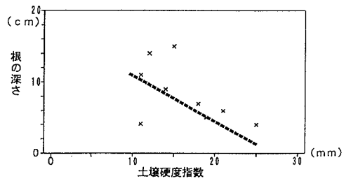
図-3 施工後4年の土壌硬度と根の深さ
