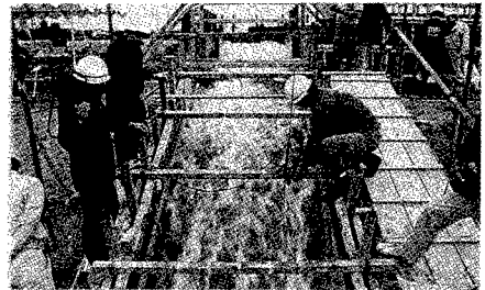
写真-1 植生の耐侵食力に関する実験状況
