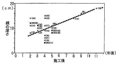
図-2 施工年数とシバの根の深さ
