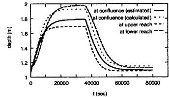
図8 水深：case(2)
