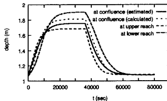
図6 水深：case(0)
