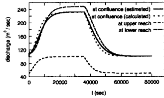
図5 流量：case(0)
