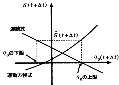
図2 q_0 の計算
