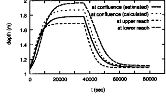
図7 水深：case(1)
