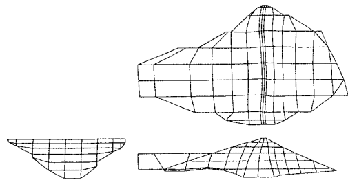
図3 上下流1次モード（3次元）
