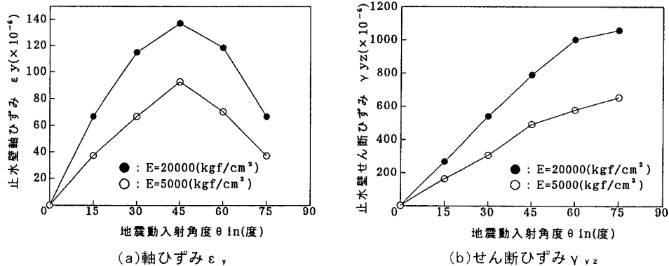
図-4 地震動入射角度 \theta_{in} と壁体最大ひずみの関係
