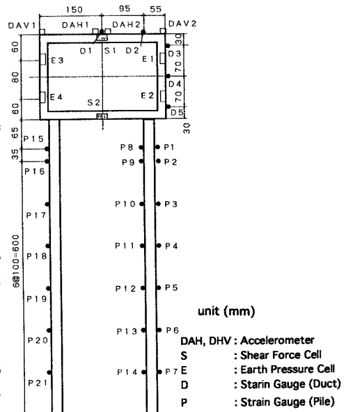
図1 洞道と杭の計測点配置
