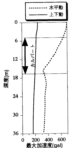
図-3 地盤の最大加速度
