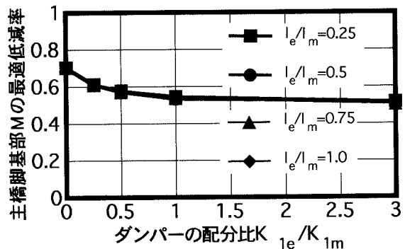
図-3 ダンパー配分比と橋脚剛性比の関係( l_m=3119\text{m}^4 )
