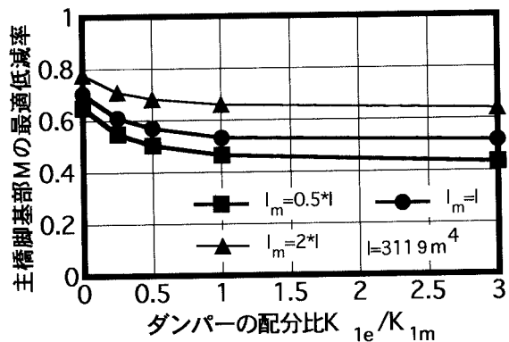
図-4 ダンパー配分比と主橋脚剛性の関係 ( l_e/l_m=0.5 )
