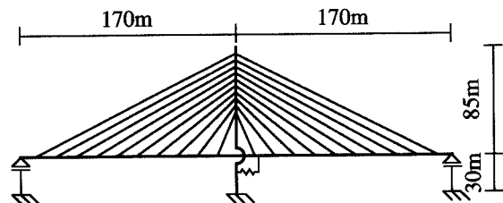
図-3 スパン170mの解析モデル
