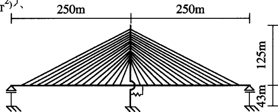
図-2 スパン250mの解析モデル
