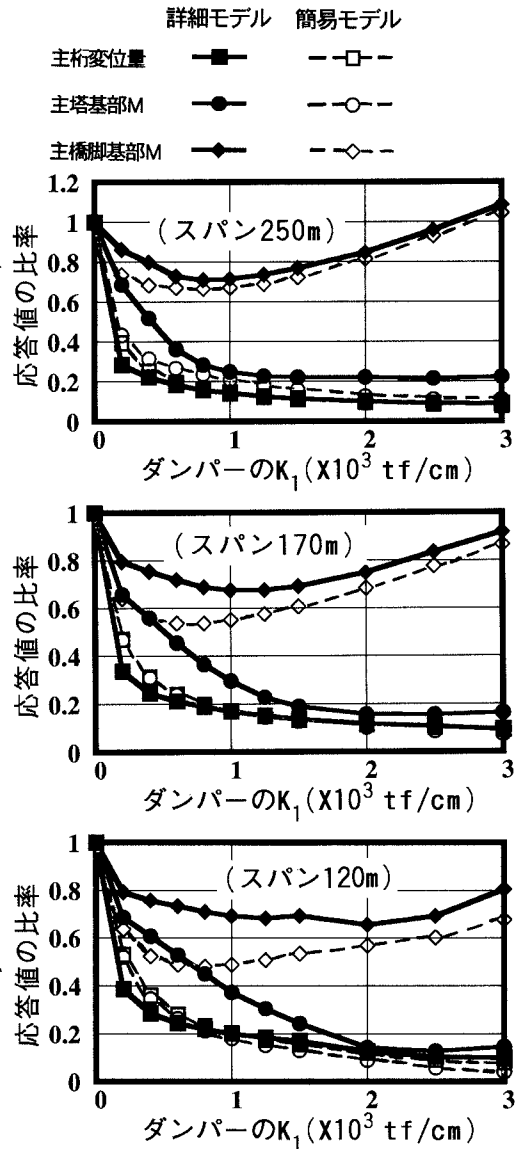
図-5 応答値の比率と K_1 の関係
