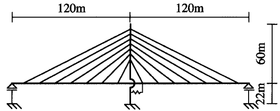
図-4 スパン120mの解析モデル
