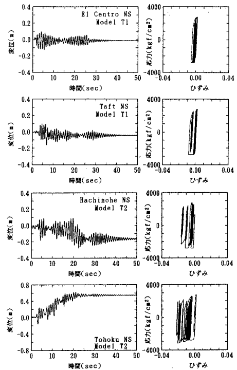
図-3 応答解析結果の一例（レベル2）
