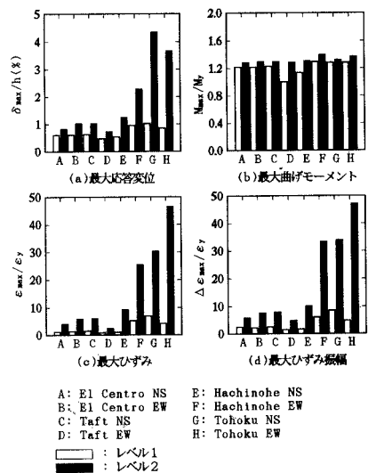
図-4 最大応答値の比較（モデルT1）
