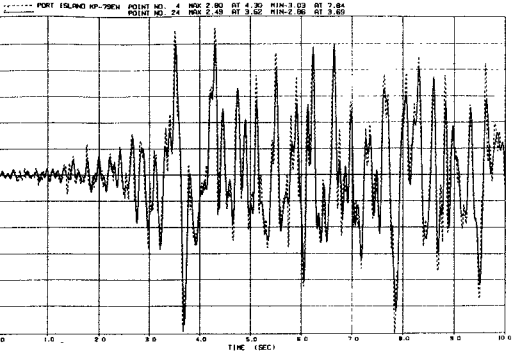
図3 観測地震波(破線)と解析波形(実線) 上からKP-0EW, 12EW, 28EW, 79EW
