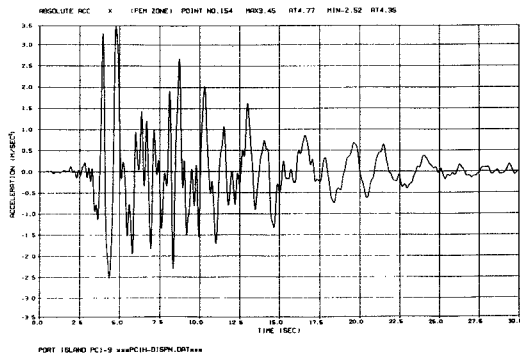
図4 海側レールの解析加速度波形
