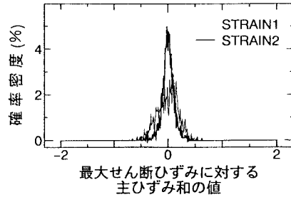
図-4 (\varepsilon_1 + \varepsilon_2) / \gamma_{max} の確率密度分布
