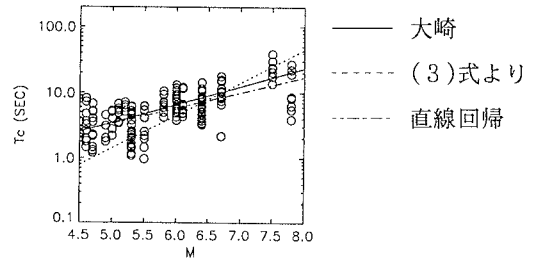
図2 M(マグニチュード)とTcの関係
