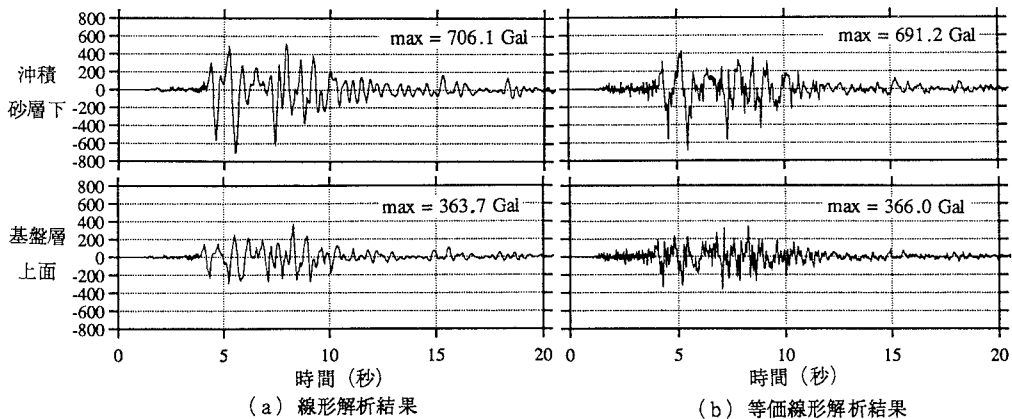
図-2 基盤層上面と沖積砂層下の加速度波形（基盤深度：150m）
