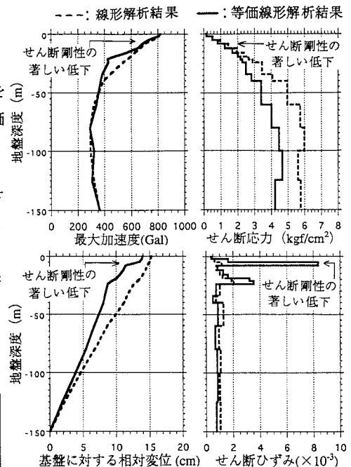
図-1 解析結果（基盤深度：150m）
