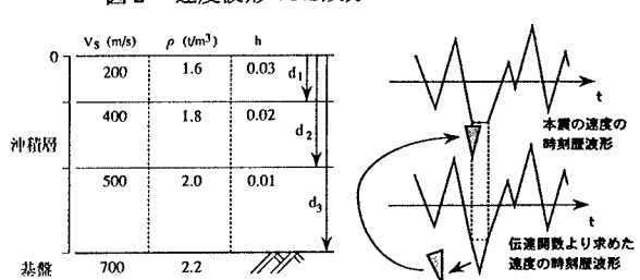
図4 地盤モデル
