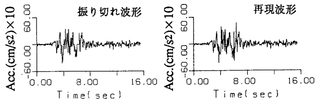
図8 加速度波形
