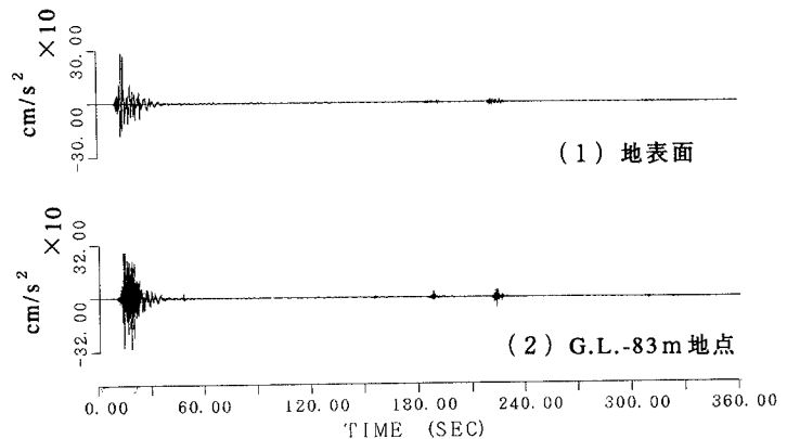
図2 観測記録（東西方向成分）
