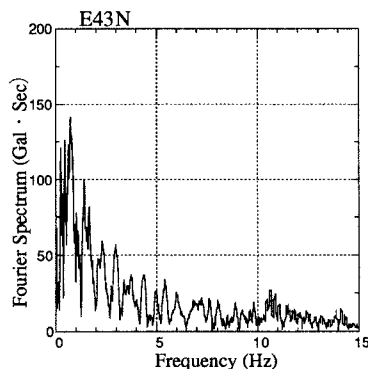
図－7 フーリエスペクトル （E 4 3 N成分）
