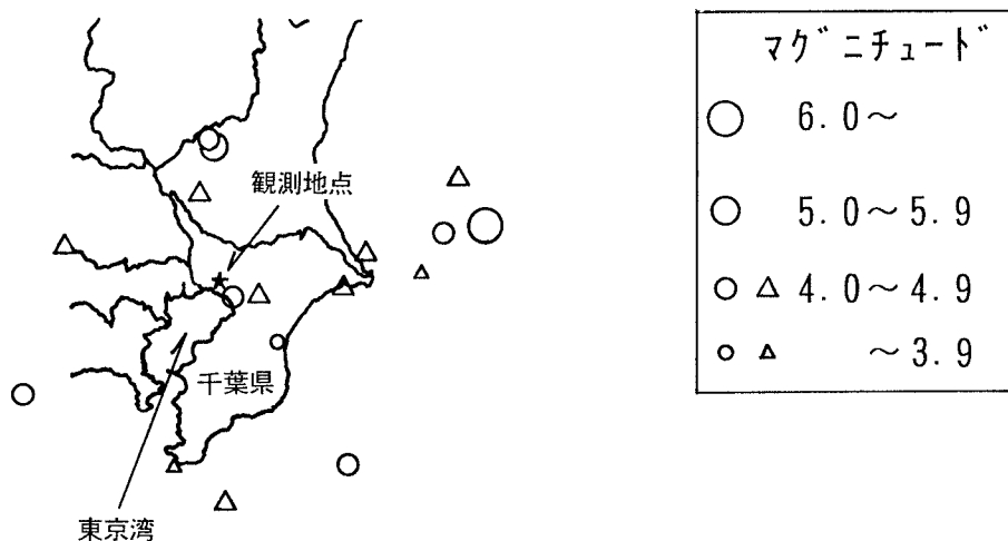
図1 震源地の位置と間隙水圧変化の有無
