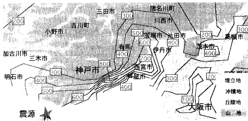
图1 最大水平加速度分布图
