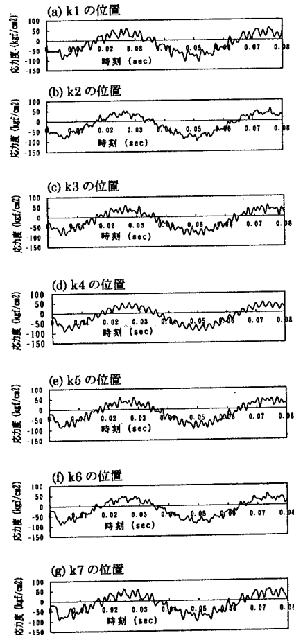
図-4 応力度の時刻歴
