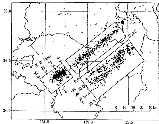
図4 余震分布
