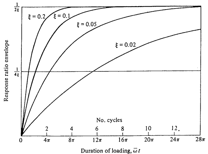
図1 正弦波による過渡的共振増幅率
