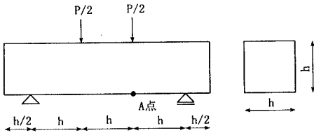
図1 はりの曲げ破壊解析モデル ( h=200\text{mm} )
