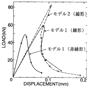
図3 荷重－変位曲線（解析結果）
