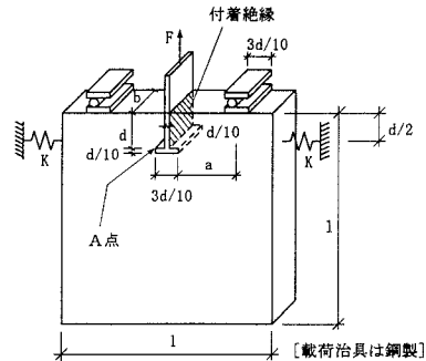
図2 アンカーボルトの引き抜き破壊解析モデル
