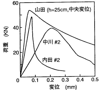
図4 荷重－変位曲線（実験結果 1) ）
