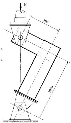
Fig. 1 Test Setup
