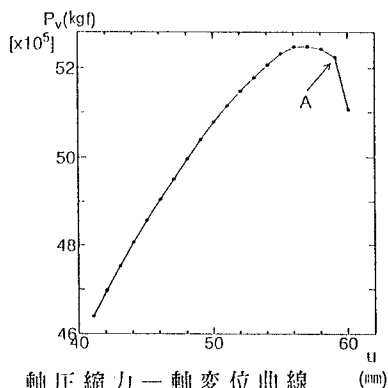
図-2 軸圧縮力-軸変位曲線
