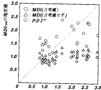
図2 MDI res -MDI関係
