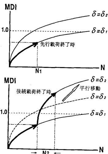
図1 MDIの計算方法
