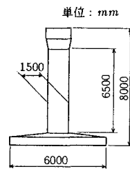
図-2: 解析対象橋脚
