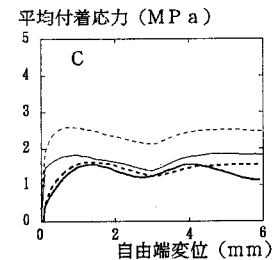
図3 平均付着応力-自由端変位曲線
