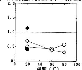
図6 指標③: 各自由端変位時の平均付着応力(健全棒材との比)
