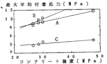
図2 最大平均付着応力とコンクリート強度の関係
