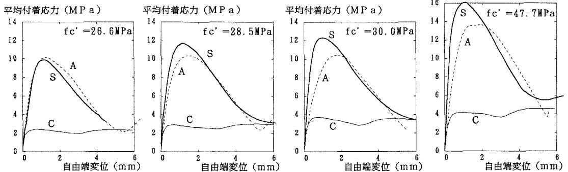
図1 平均付着応力-自由端変位曲線（健全棒材、コンクリート強度別）
