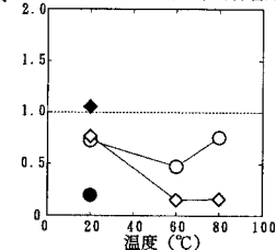
図6 指標③: 各自由端変位時の平均付着応力(健全棒材との比)
