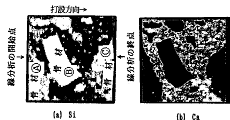
写真1 コンクリート中のSi, Caの分布 (W/C:0.60, 湿潤養生14日)
