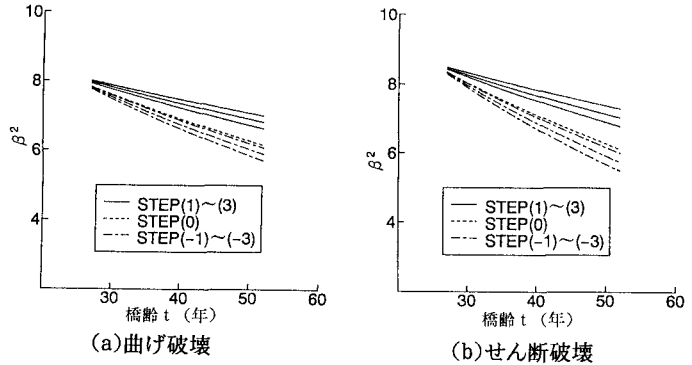
図2 主桁間剛性比の変動による安全性の変化
