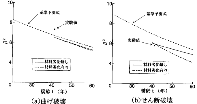
図3 安全性評価結果
