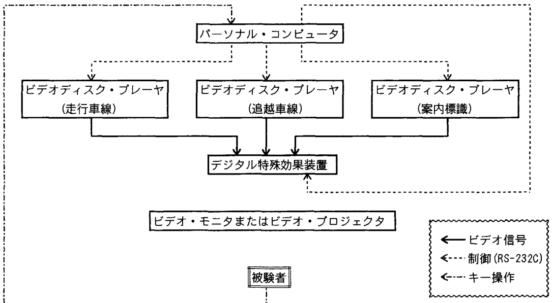
図-1 簡易走行模擬装置の構成
