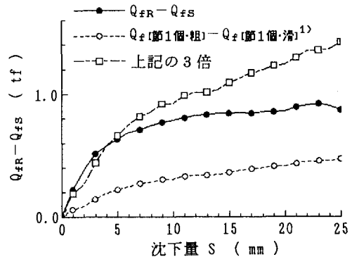
図-4 (Q_{RR}-Q_{RS}) -沈下量関係
