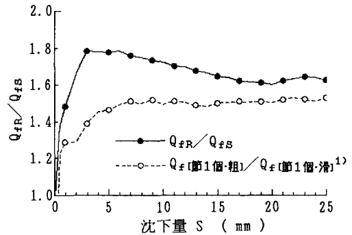
図-3 (Q_{RR}/Q_{RS}) -沈下量関係
