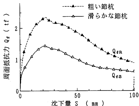
図-2 周面抵抗 Q_r -沈下量(S)関係
