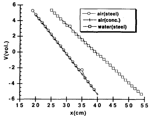
図-3 水中および空気中での較正結果
