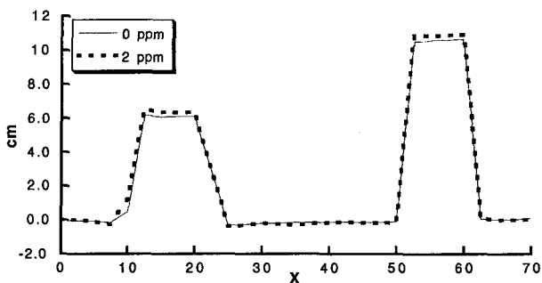
図-6 濁水中での底面形状の測定結果
