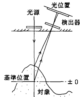
図-1 レーザー光による測定原理
