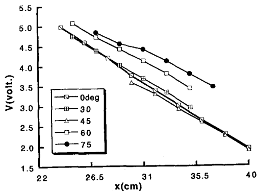
図-4 傾斜面に対する距離測定
